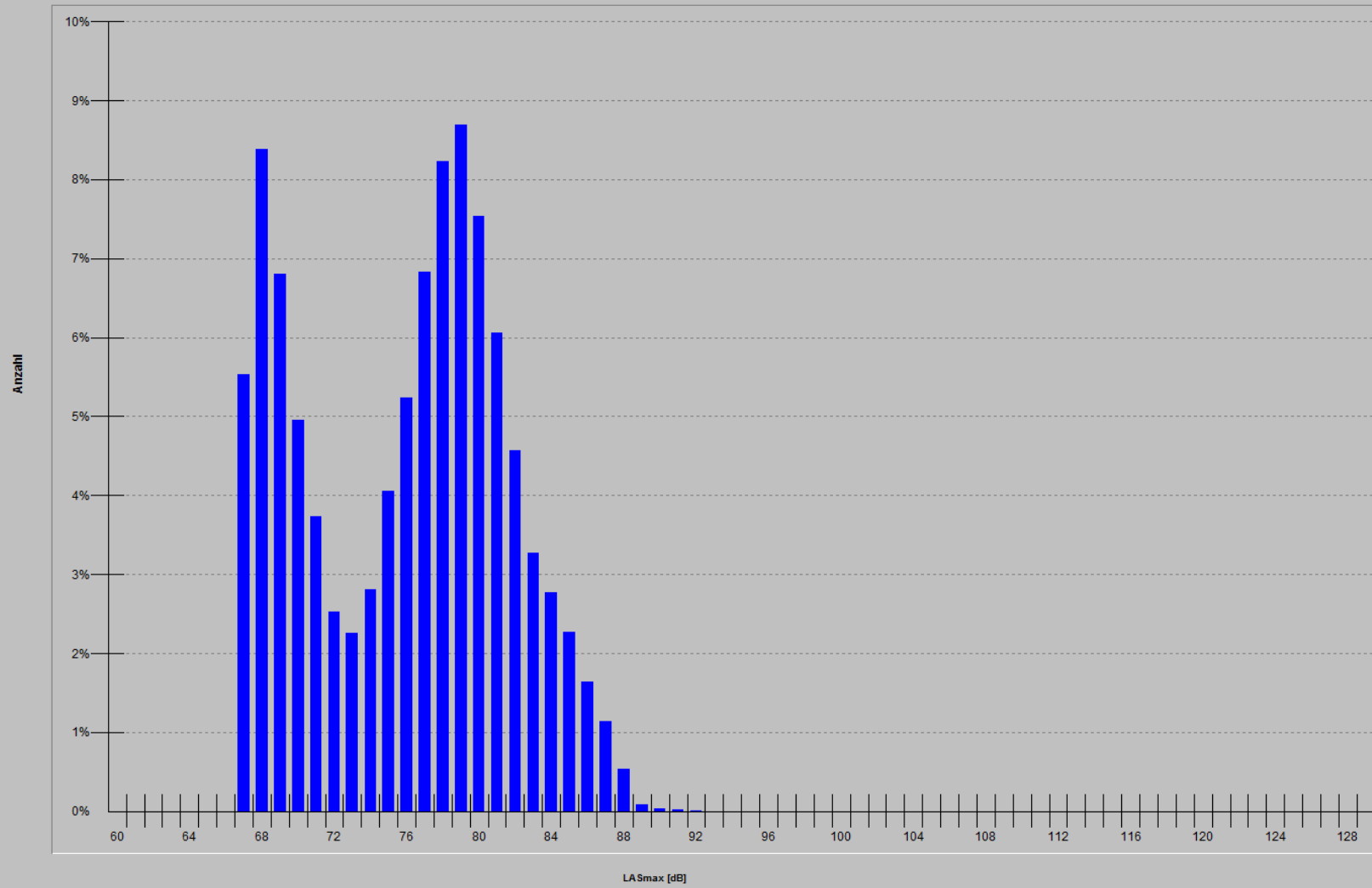
Maximalpegel-Verteilung korr. Lärmereignisse MP08 2018
