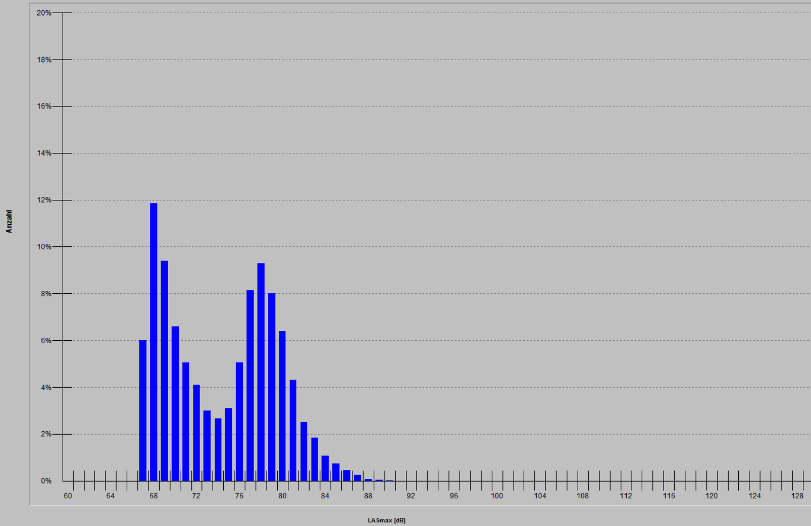
Maximalpegel-Verteilung korr. Lärmereignisse MP01 2018
