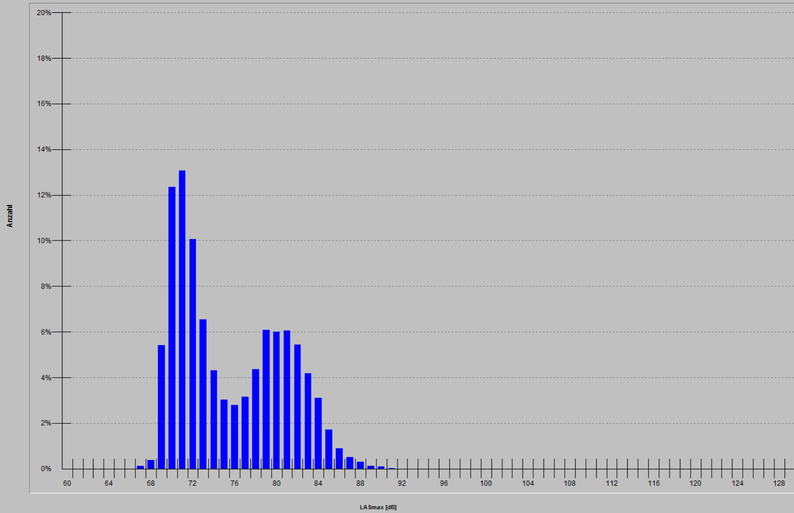
Maximalpegel-Verteilung korr. Lärmereignisse MP02 2018
