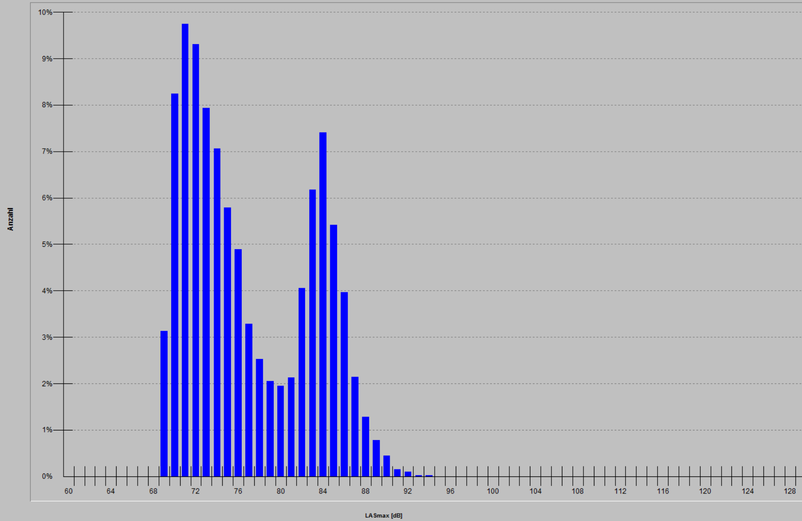
Maximalpegel-Verteilung korr. Lärmereignisse MP05 2018
