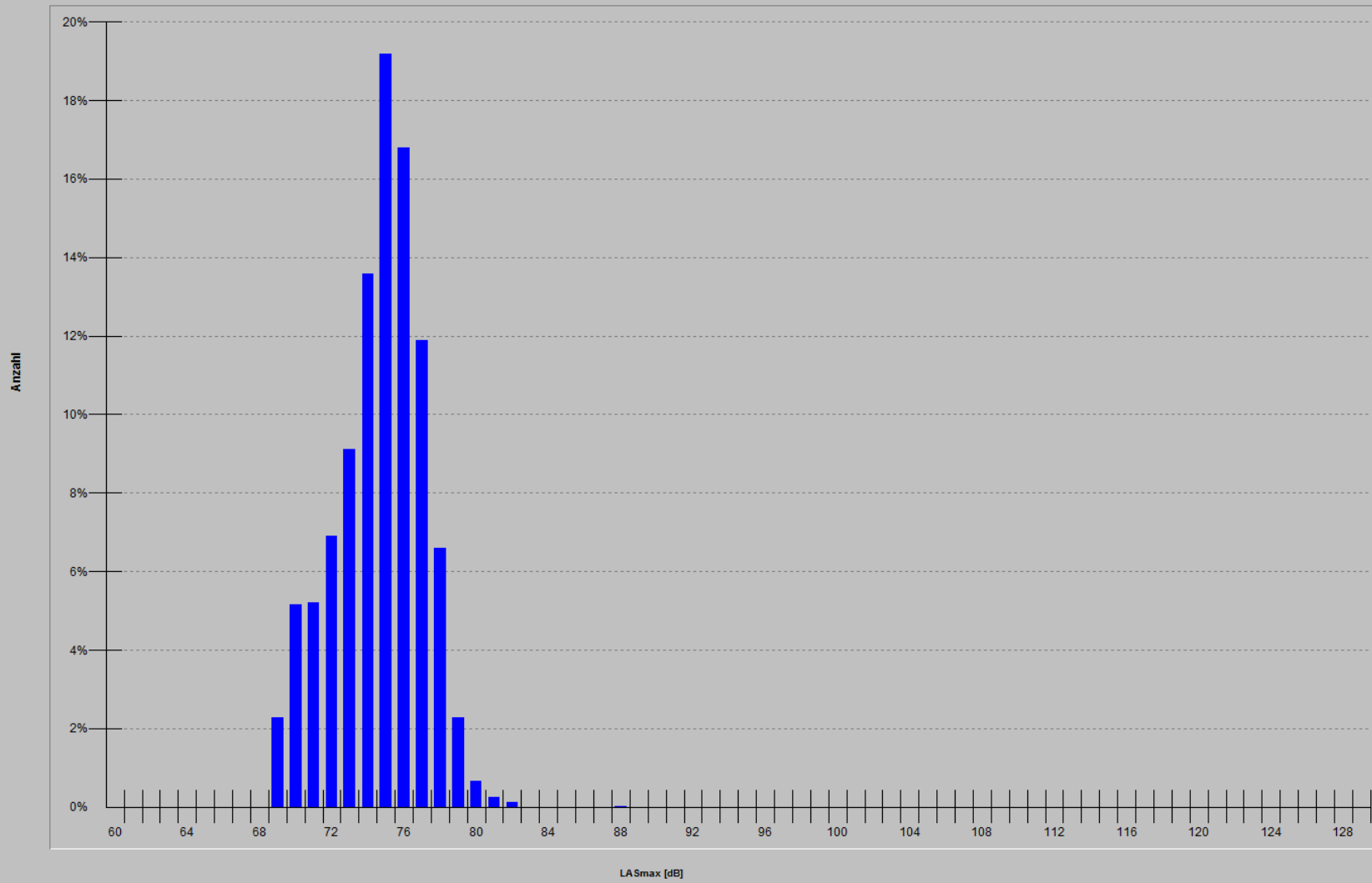
Maximalpegel-Verteilung korr. Lärmereignisse MP10 2018
