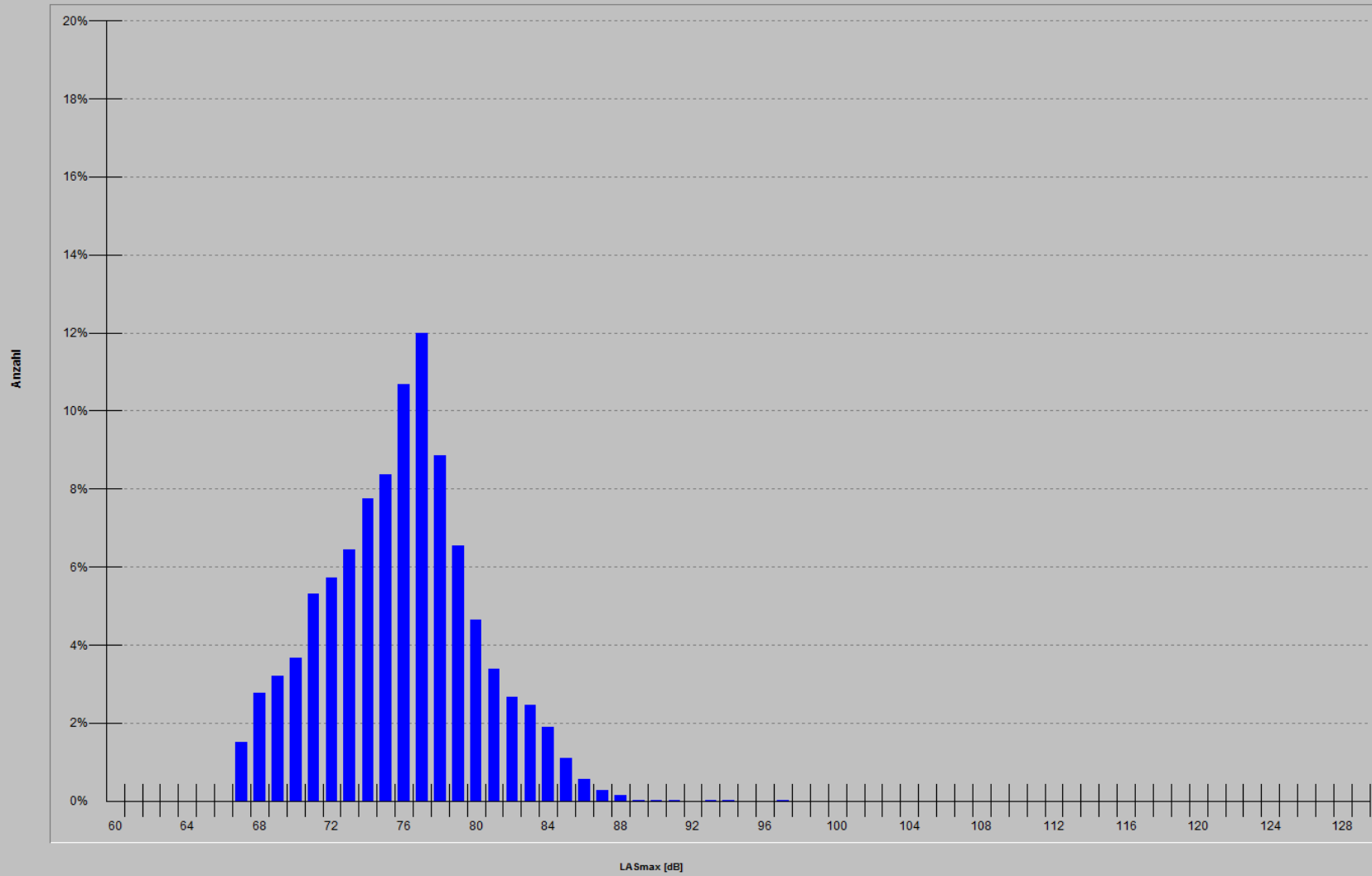
Maximalpegel-Verteilung korr. Lärmereignisse MP07 2018
