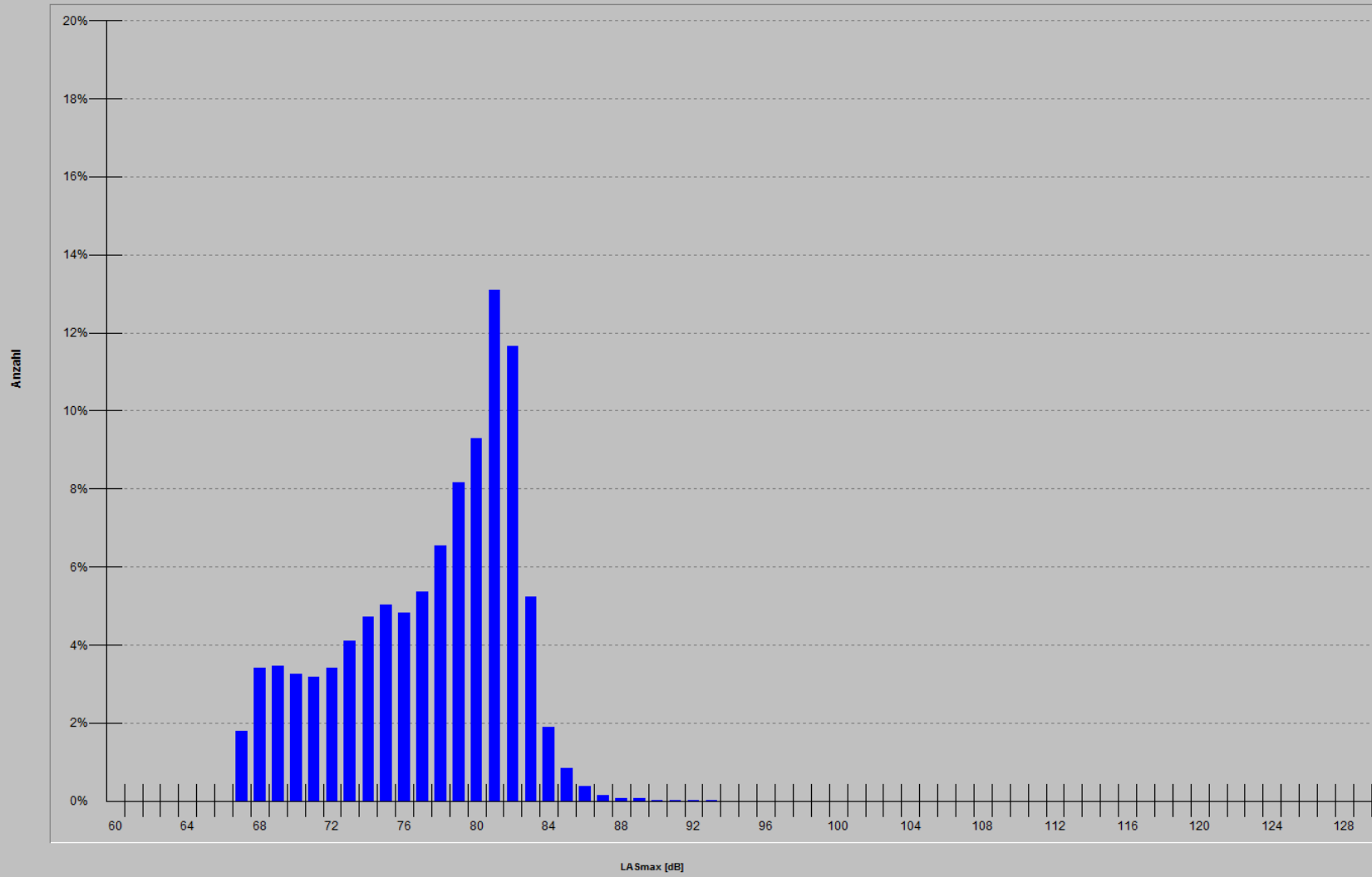
Maximalpegel-Verteilung korr. Lärmereignisse MP09 2018
