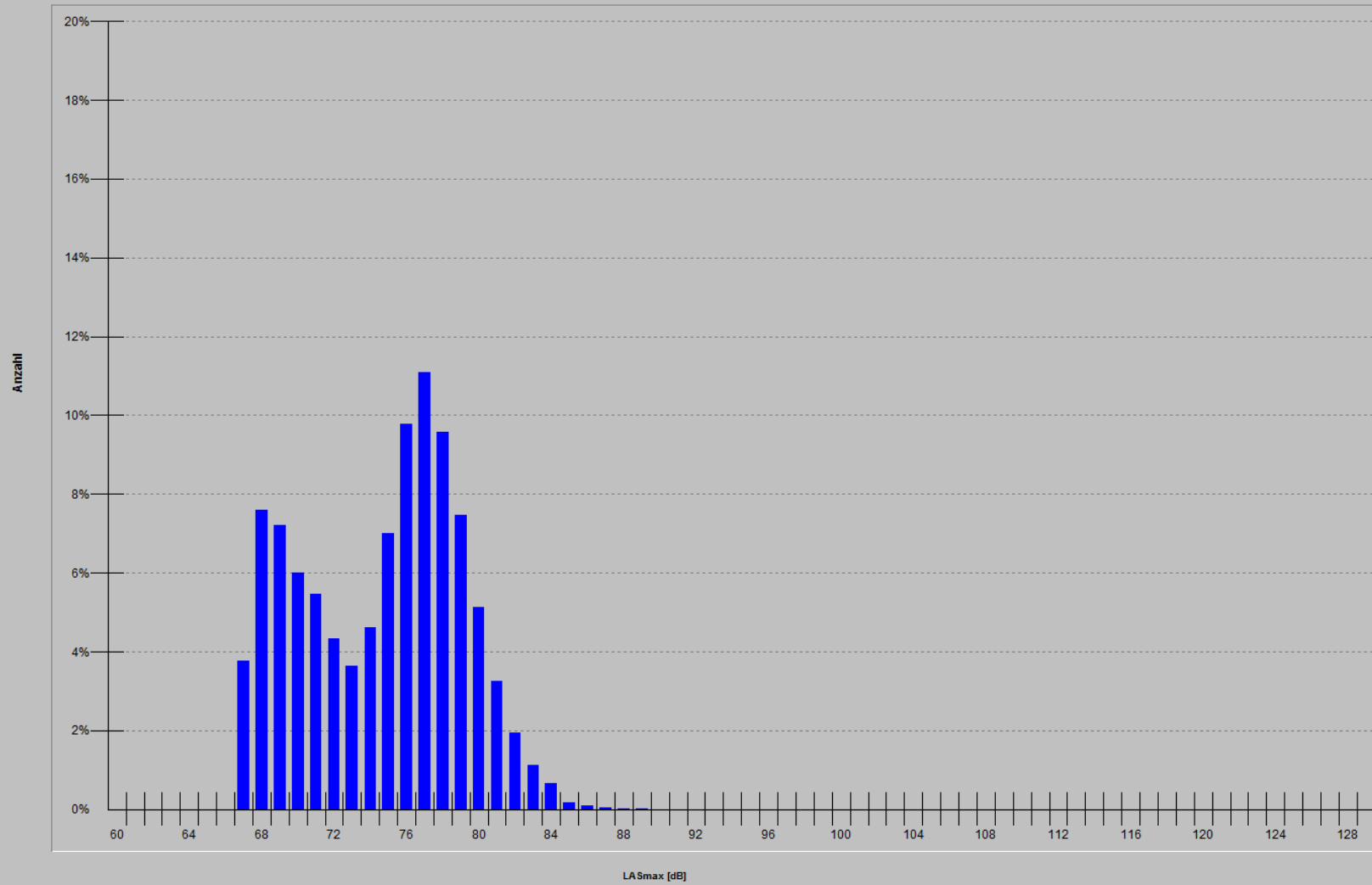
Maximalpegel-Verteilung korr. Lärmereignisse MP06 2018
