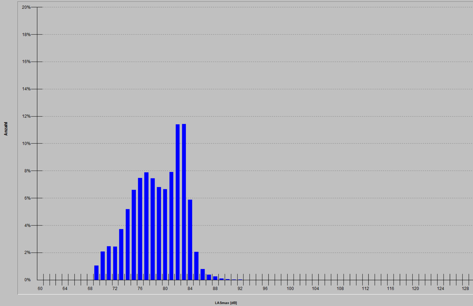
Maximalpegel-Verteilung korr. Lärmereignisse MP04 2018
